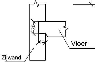
Aansluiting vloer en zijwand
